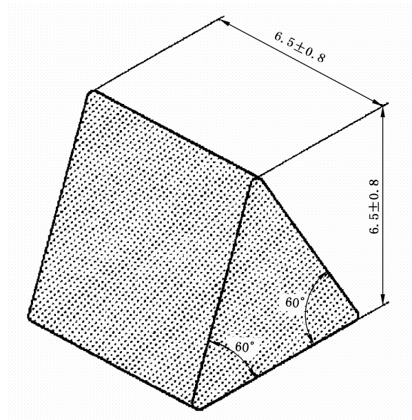
图 C.3 试验块
